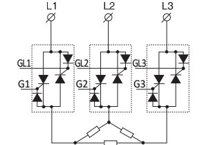
AIJK-33 角型三相三线全控制结构 (单向可控硅反并联电路，推荐采用 MCC 系列功率模块)
