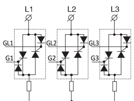
AIJK-33 星型三相三线全控制结构 (单向可控硅反并联电路，推荐采用 MCC 系列功率模块)
