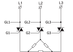
AIJK-33 角型三相三线全控制结构 (双向可控硅电路)
