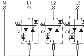
AIJK-30 星型三相四线制结构负载 (单向可控硅反并联电路，推荐采用 MCC 系列功率模块)
