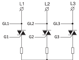
AIJK-33 星型三相三线全控制结构 (双向可控硅电路)
